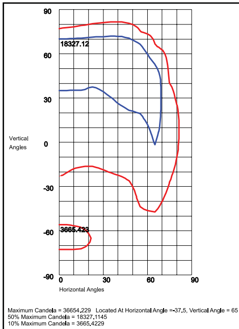
FXKH55QD2X256U5KC 110°H x 30°V, NEMA 6H x 5V
