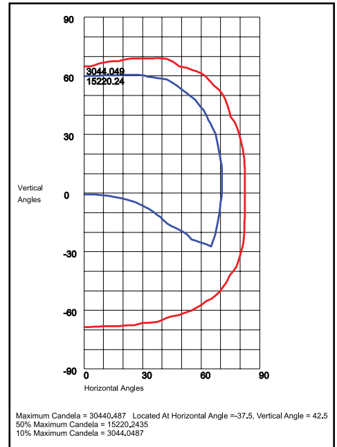
FXKH55QC2X256U5KC 120°H x 70°V, NEMA 7H x 7V
