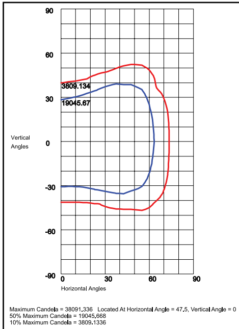
FXKH55QA2X256U5KC 130°H x 70°V, NEMA 7H x 5V
