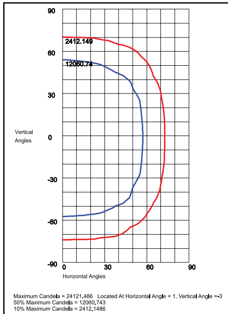
FXKH55QF2X256U5KC 110°H x 110°V, NEMA 7H x 7V
