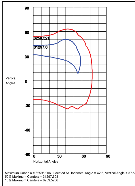
FXKH55QB2X256U5KC 110°H x 30°V, NEMA 7H x 6V
